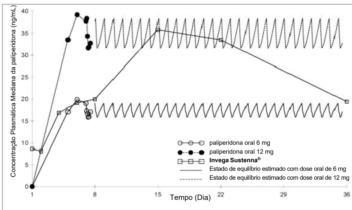
Figura 4 . Perfis de concentração plasmática mediana versus tempo seguindo os perfis farmacocinéticos medianos da paliperidona por 5 semanas após a administração do Invega Sustenna® utilizando o esquema de iniciação recomendado (iniciando com palmitato de paliperidona equivalente a paliperidona 150 mg/100 mg no músculo deltoide nos dia 1/dia 8) em comparação à administração diária de um comprimido oral de liberação prolongada (6 mg ou 12 mg).
